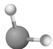
molécula de agua
