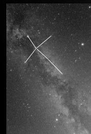
La Vía Láctea con la figura de la Cruz del Norte en Cisne
