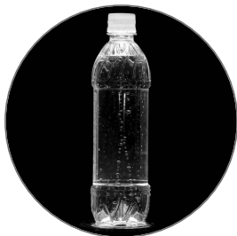
33,000,000,000,000,000,000,000,000 (33 trillones de trillones) de moléculas de agua
