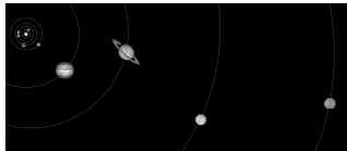
Este diagrama muestra los planetas moviéndose alrededor del sol en nuestro sistema solar.
